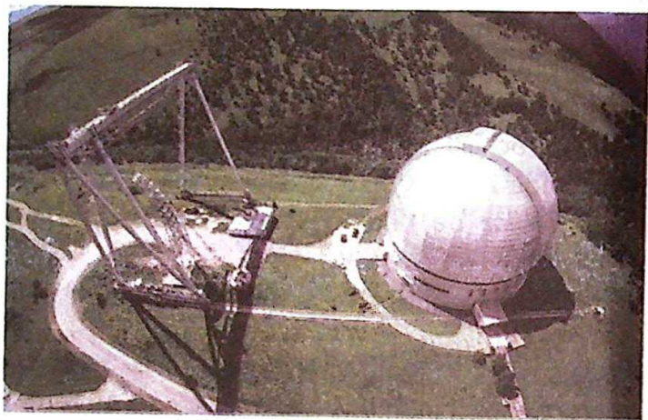
37-rasm. Shimoliy Kavkazdagi ko'zgusining diametri 6 metrli teleskop-reflektor minorasining ko'rinishi.
