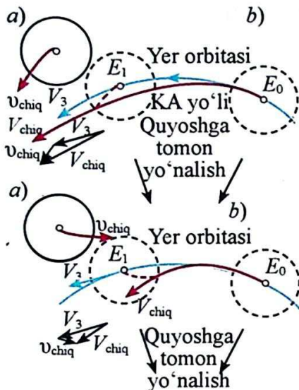
124-rasm. KANing Yer ta'sir sferasidagi harakati: a va b (yuqorida) – tashqi planetalarga uchish; a va b (pastda) – ichki planetalarga uchish sxemalari; a ) geosentrik; b ) geliosentrik trayektoriyalar.
