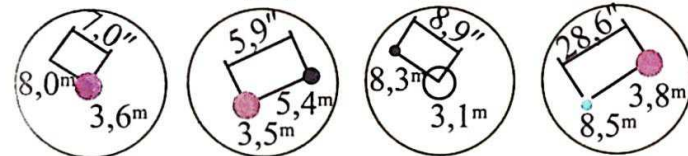
Javzonning \kappa si Gerkulesning \alpha si Gerkulesning \delta si Perseyning \eta si
