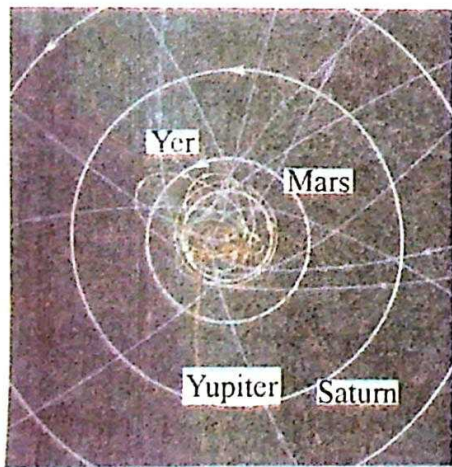
84-rasm. Kometalardan bir guruhining Quyosh atrofidagi orbitalari.
