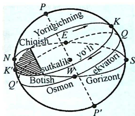
13-rasm. Yoritgichlarning kulminatsiya hodisasi.
