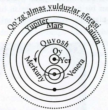
25-rasm. Beruniyning olam tuzilishi haqidagi qarashlariga ko‘ra, Quyosh o‘z atrofida aylanayotgan yo‘ldoshlari – Merkuriy va Venera bilan birga Yer atrofida aylanadi.
