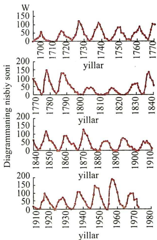
54-rasm. Quyosh aktivligining (dog'lari sonining yillar bo'ylab) o'zgarish grafigi.
