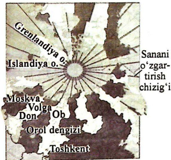
16-rasm. Yer shari poyaslari.
