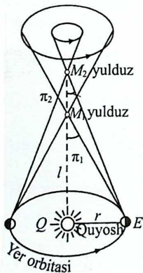
90-rasm. Yulduzlarning yillik parallaksi.
