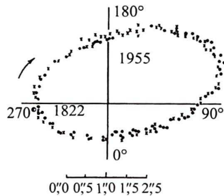
95-rasm. Vizual qo'shaloq yulduz (Katta Ayiqlning \xi yulduzi) orbitasi.
