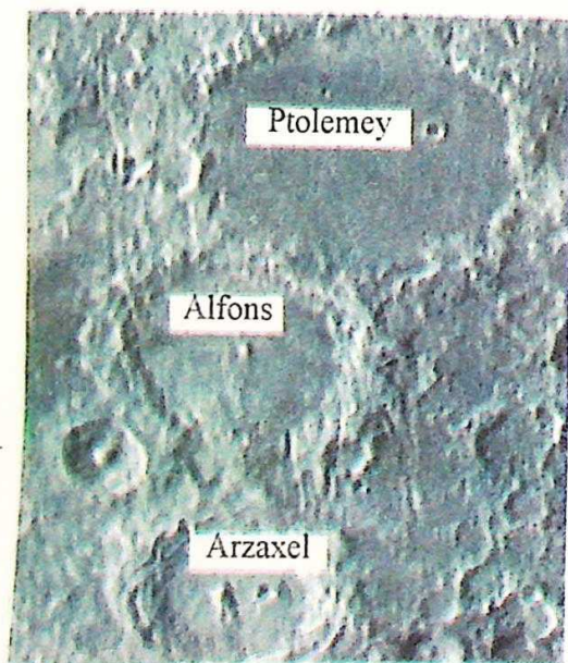
63-rasm. Oy kraterlari va «dengizlari».
