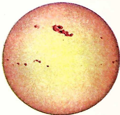
46-rasm. Quyosh fotosferasi (dog'lari bilan).
