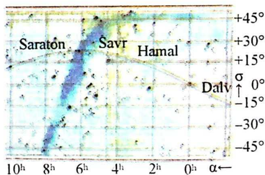
9-rasm. Yulduz xaritasi.
