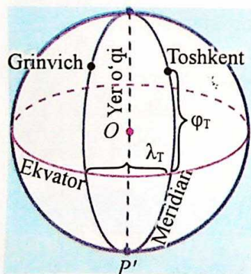
7-rasm. Geografik koordinatalar sistemasi.
