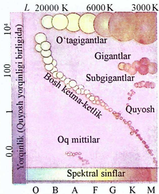
93-rasm. Spektr-yorqinlik diagrammasi.
