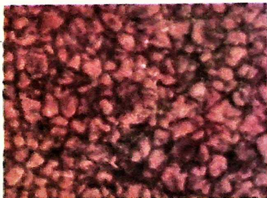
47-rasm. Quyosh sirtining haqiqiy strukturasi – donadorlik (granulatsiya).
