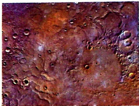
57-rasm. Merkuriy sirtining relyefi.
