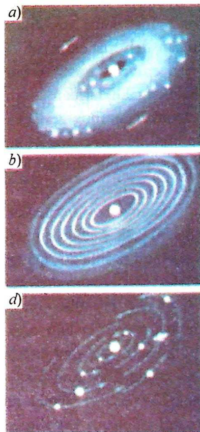
89-rasm. Quyosh sistemasining paydo bo'lishi.
