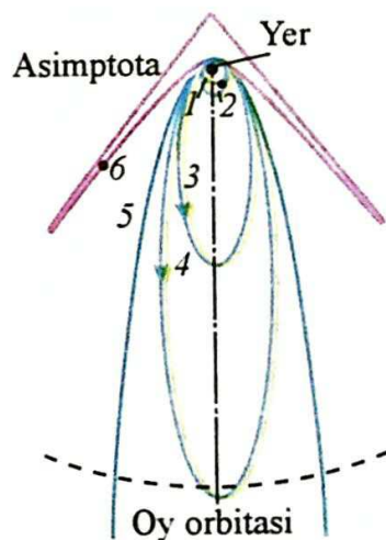
33-rasm. Yer tortishish maydonida jismlarning harakat trayektoriyalari.
