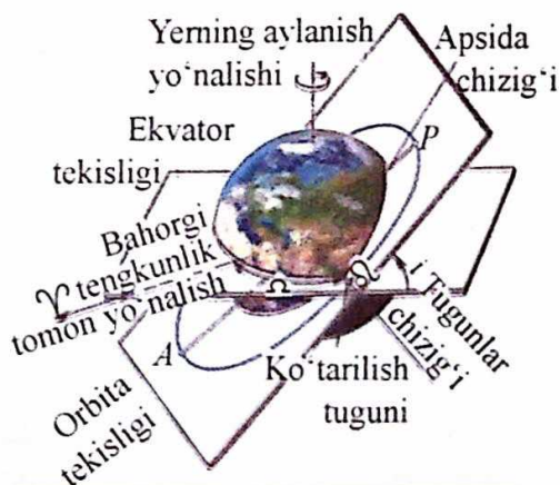
118-rasm. Sun'iy yo'ldoshning orbita elementlari.
