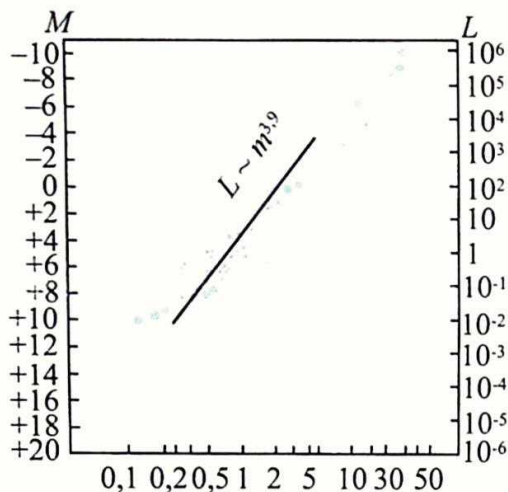
97-rasm. Yulduzlarning yorqinliklari va massalari orasidagi bog‘lanish.
