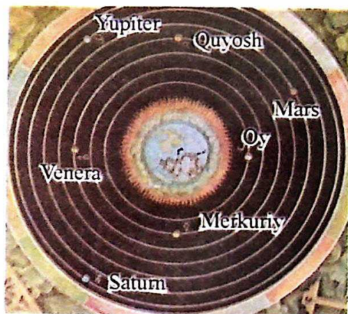
1-rasm. Aristotel (mil. avv. IV asr) Olam tuzilishini shunday tasavvur qilgan.
