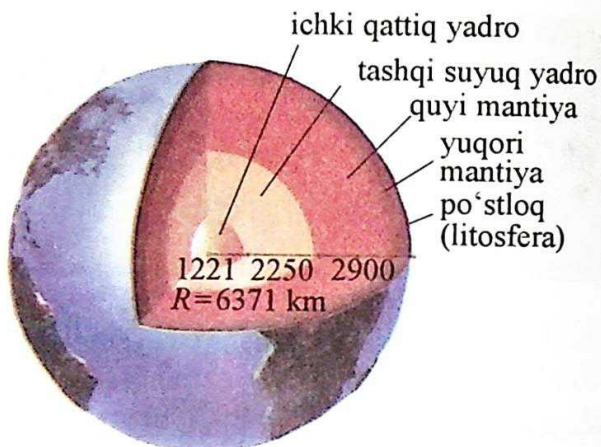
60-rasm. Yerning ichki tuzilishi.
