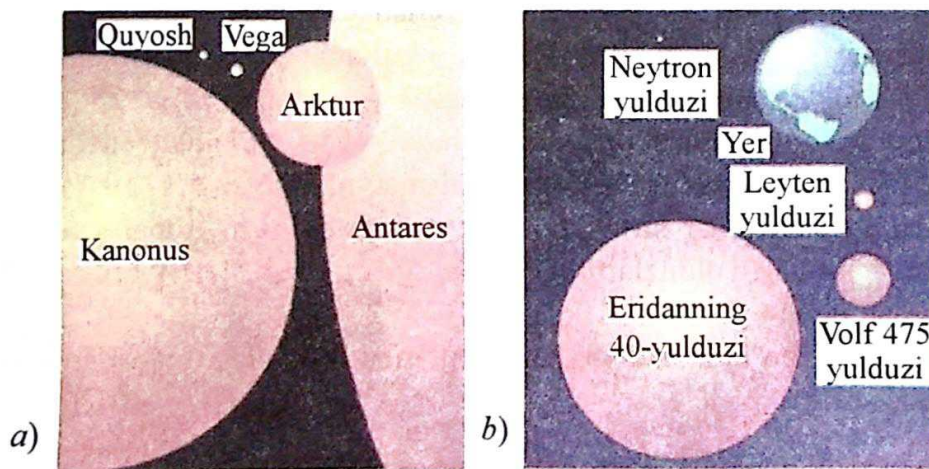
91-rasm. Quyosh o'lchami gigant yulduzlar (a) Yer o'lchami kattaligidagi mitti yulduzlar (b) bilan solishtirilgan.
