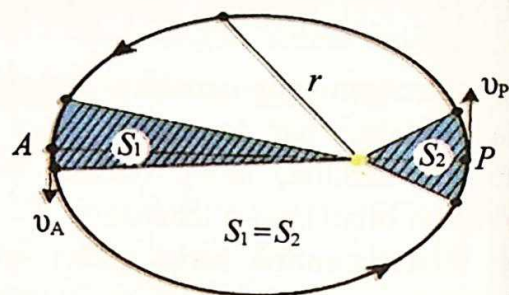
32-rasm. Planeta radius-vektorlarining teng vaqtlarda chizgan teng yuzalari.
