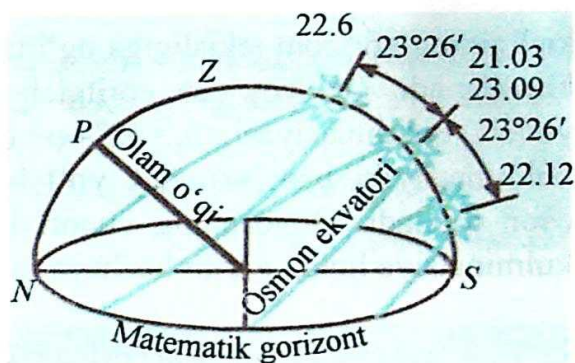
12-rasm. Yil davomida, tush paytida Quyosh balandligining o'zgarishi.
