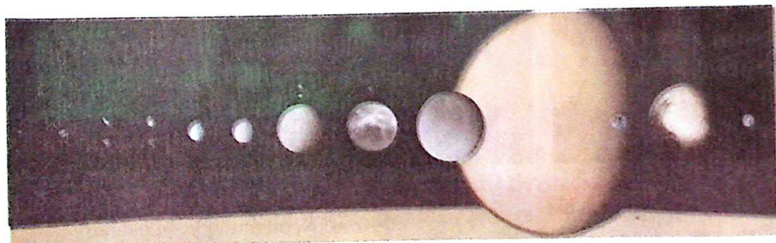
77-rasm. Saturnning yo'ldoshlari (eng yirigi – Titan).
