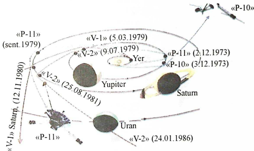
74-rasm. «Pioner-10», «Pioner-11» («P-10», «P-11») va «Voyajer-1», «Voyajer-2» («V-1», «V-2»)larning trayektoriyalari.
