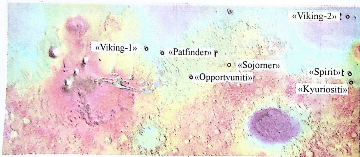
66-rasm. Marsning Ellada, Tarsis va Argir pasttekisliklari vohasining xaritasi (rasmda bu pasttekisliklarga qo'ngan kosmik apparatlarning nomlari ko'rsatilgan).
