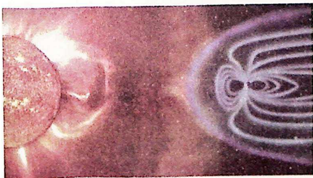
61-rasm. Yer magnitosferasining strukturasi.
