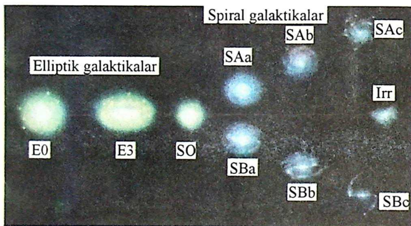
III-rasm. Galaktikalarning evolutsiyasi.
