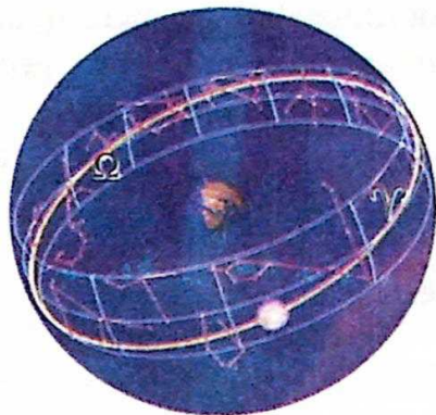
6-rasm. Ekliptika tekisligi bo'ylab joylashgan yulduz turkumlari – zodiak soha.
