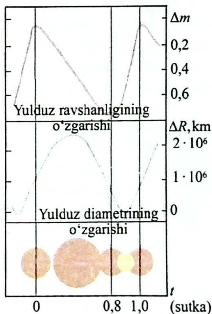
98-rasm. Sefeid (Sefeyning \delta tipidagi yulduz)larning ravshanligi ( \Delta m ) va radiusining o'zgarish ( \Delta R ) egriliklari.
