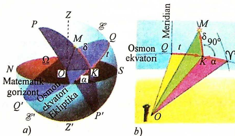
8-rasm. Ekvatorial koordinatalar sistemasi.
