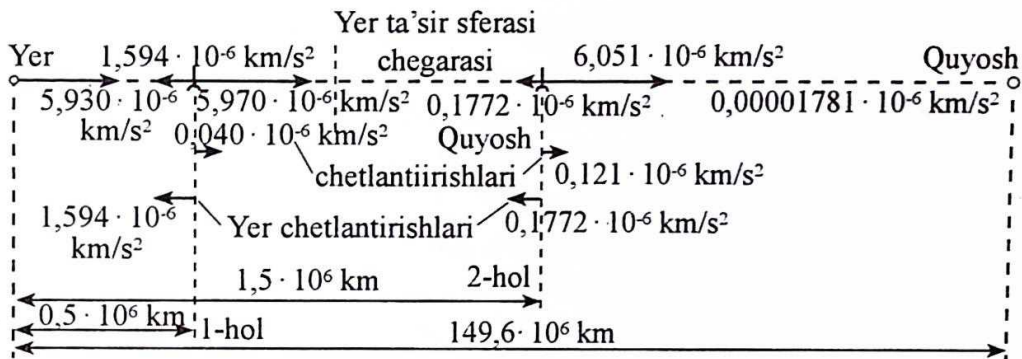
117-rasm. Yerdan va Quyoshdan berilayotgan chetlanishlarni hisoblash.
