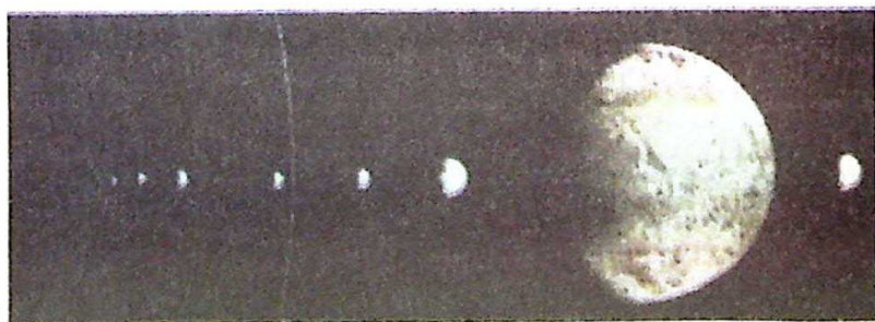
80-rasm. Neptunning yoʻldoshlari (eng yirik yoʻldoshi – Triton).
