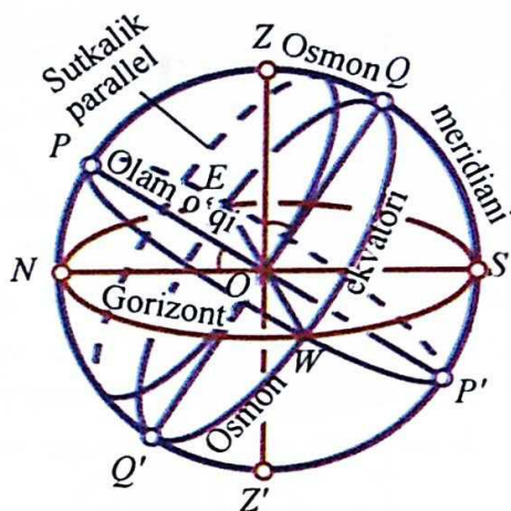
4-rasm. Osmon sferasining asosiy nuqta, chiziq va aylanalari.
