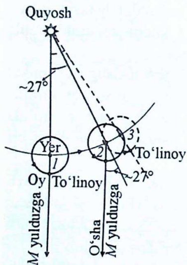
18-rasm. Oyning Yer atrofida aylanish siderik va sinodik davrlarini tushuntirish.
