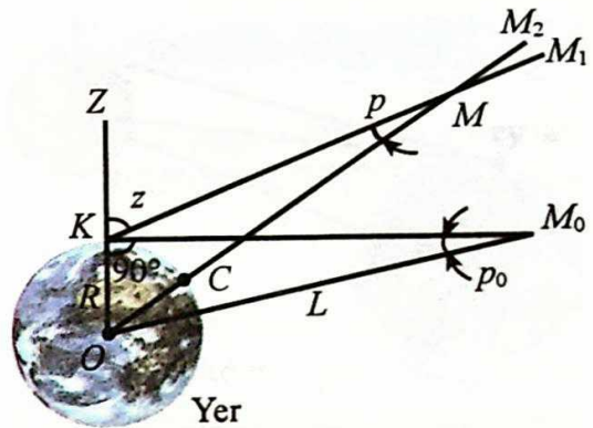
29-rasm. Yoritgichlarning sutkalik ( p ) va sutkalik gorizontal ( p_0 ) parallaksi.
