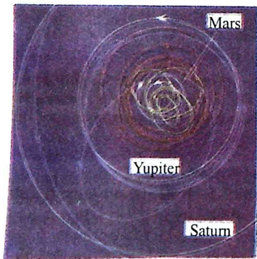
81-rasm. Bir guruh mayda planetalarning orbitalari.
