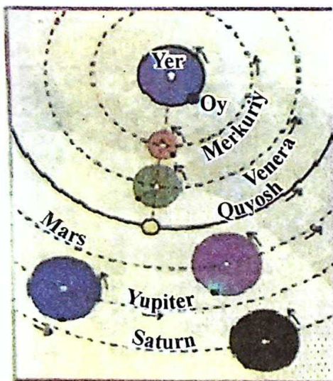
22-rasm. Ptolemeyning geosentrik sistemasi.
