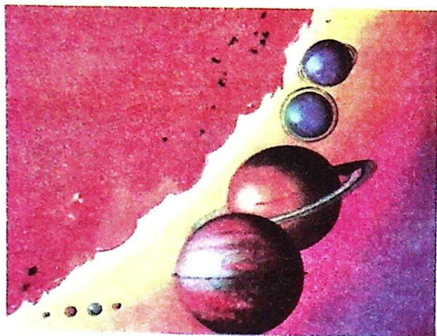
44-rasm. Quyoshning planetalar bilan solishtirilgan o'lchami.
