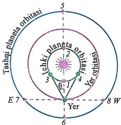
28-rasm. Planetalarning konfiguratsiyalari va ko'rinish shartlari.
