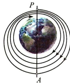
120-rasm. Yer atmosferasida sun'iy yo'ldoshning tushishi: tushish orbitalarining ko'rinishi.
